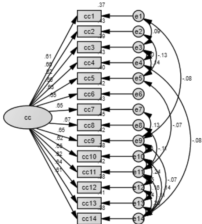
Model_cc
